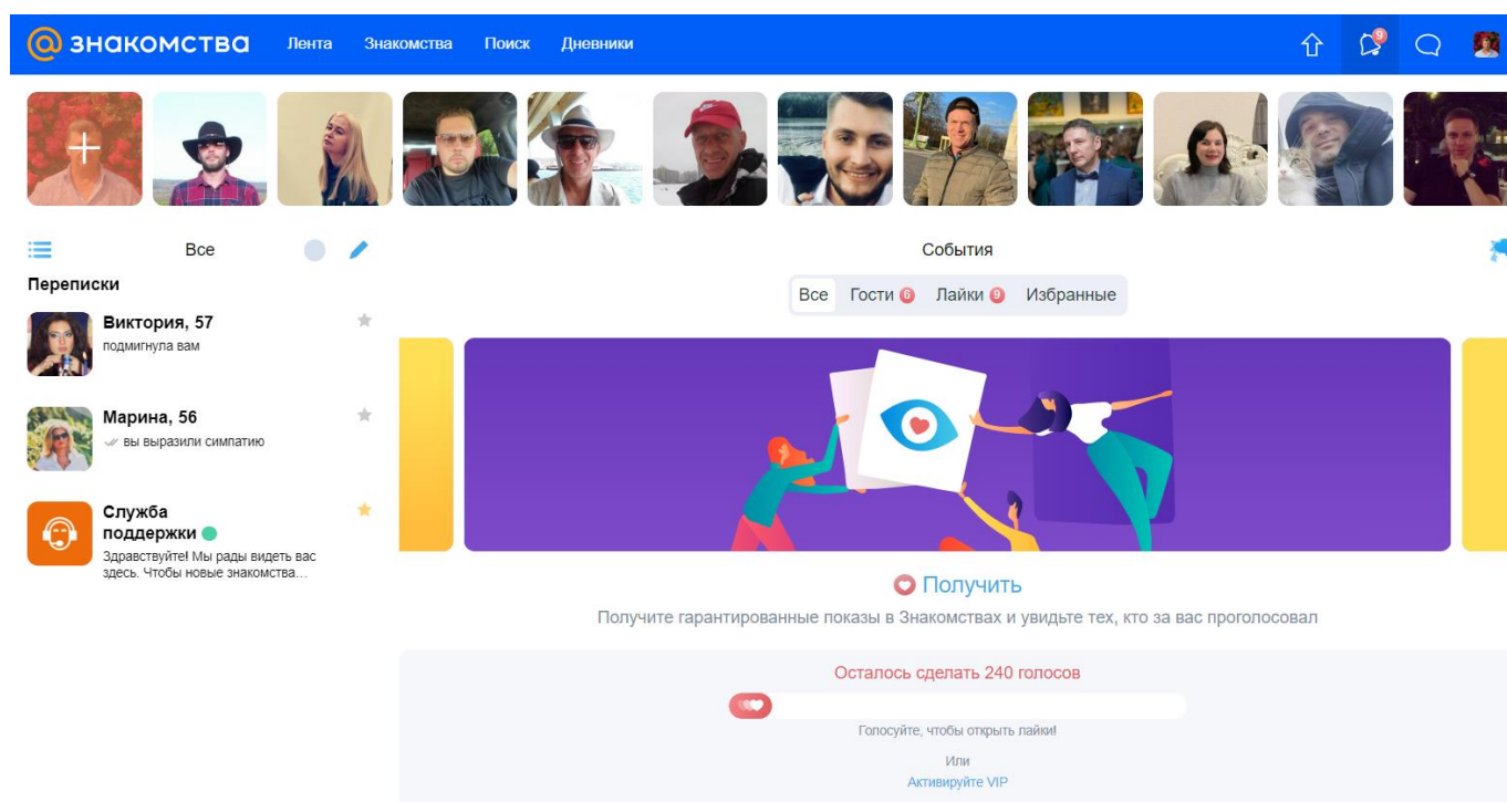
Рисунок 6 – Экран событий
